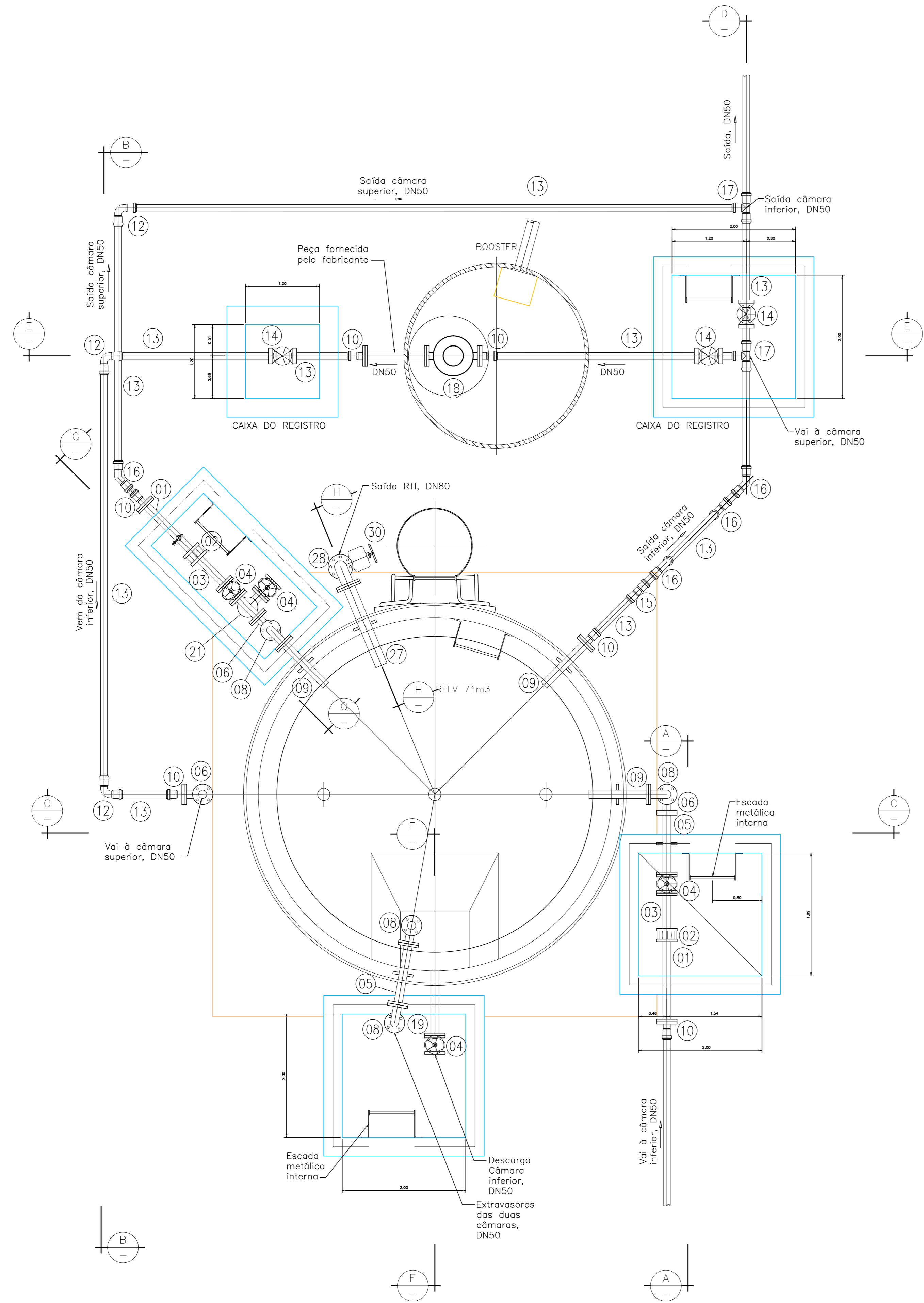
PLANTA NÍVEL RESERVATÓRIO INFERIOR - ESC. 1:25
